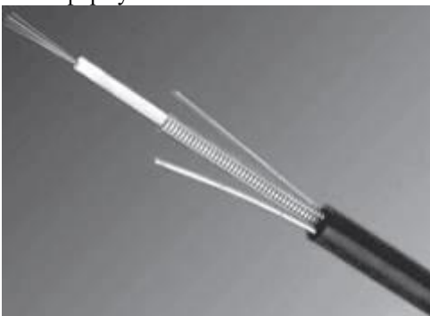
Рис. 5. Оптоволоконный кабель
