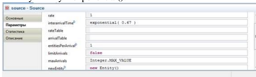
Рис. 3.8. Задание закона распределения потока заявок.
