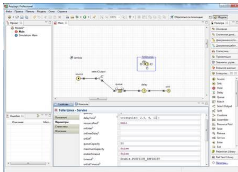
Рис. 3.23. Задание свойств линии касс.
