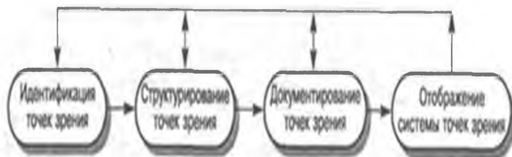
Рисунок 3 – Метод VORD
