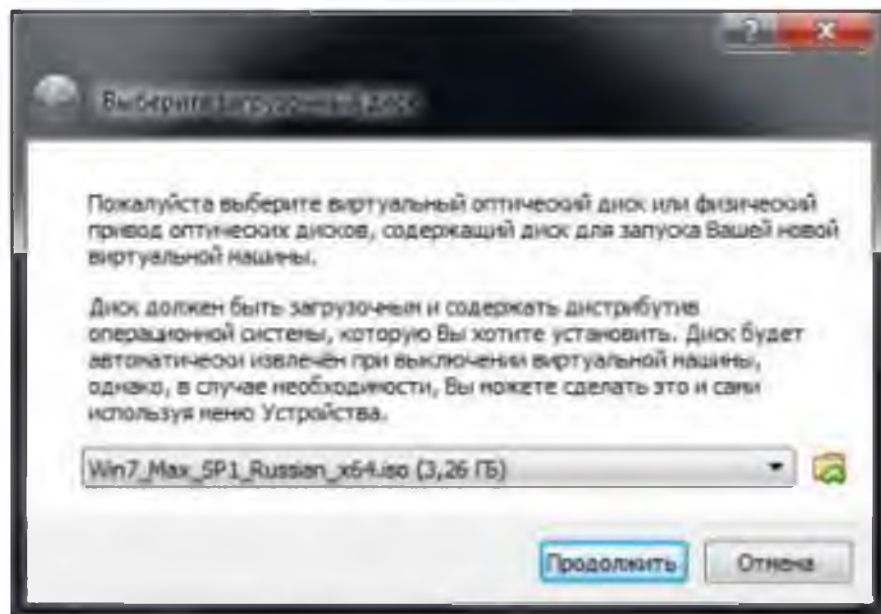
Рисунок 8 – выбор образа
